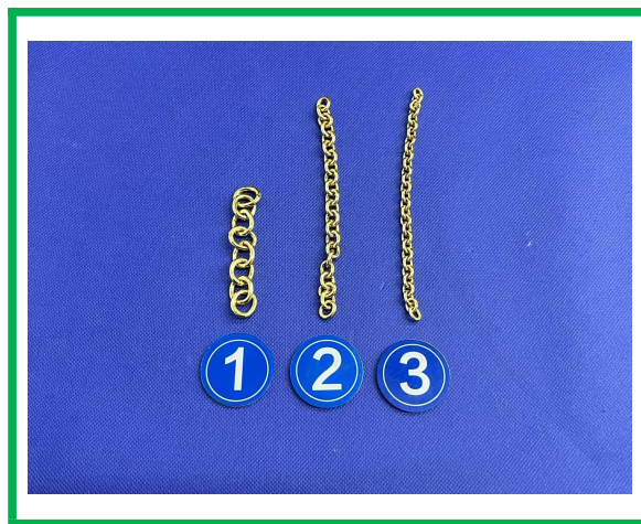
盐雾测试后
